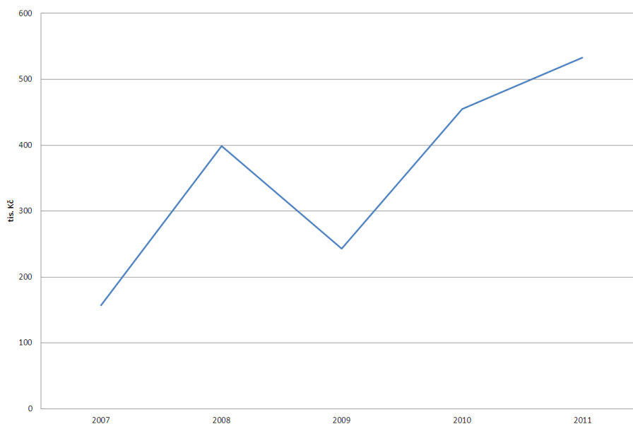
Graf 4: Vývoj hospodářského výsledku v letech 2007 – 2011
